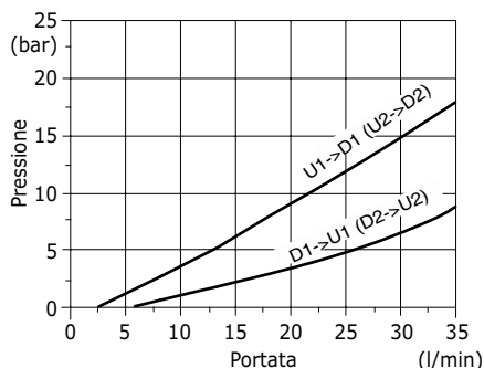
Diagramma perdite di carico VABAL 12 U1->D1 (U2->D2) e D1->U1 (D2->U2)
