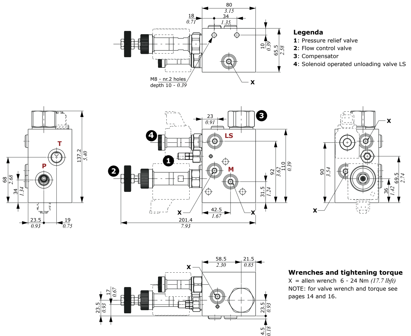
AN14 type for Open Center circuit
